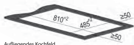
Aufliegendes Kochfeld
