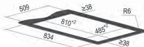
Flächenbündiges Kochfeld
